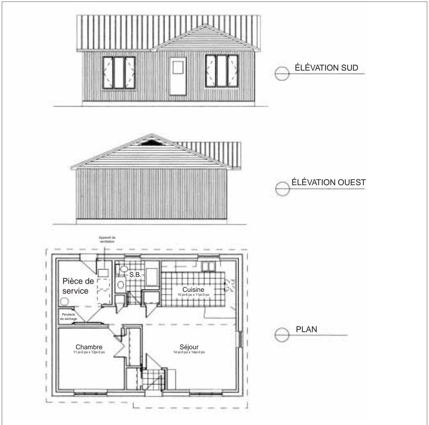
Figure 1 : Élévations et plan de la maison
