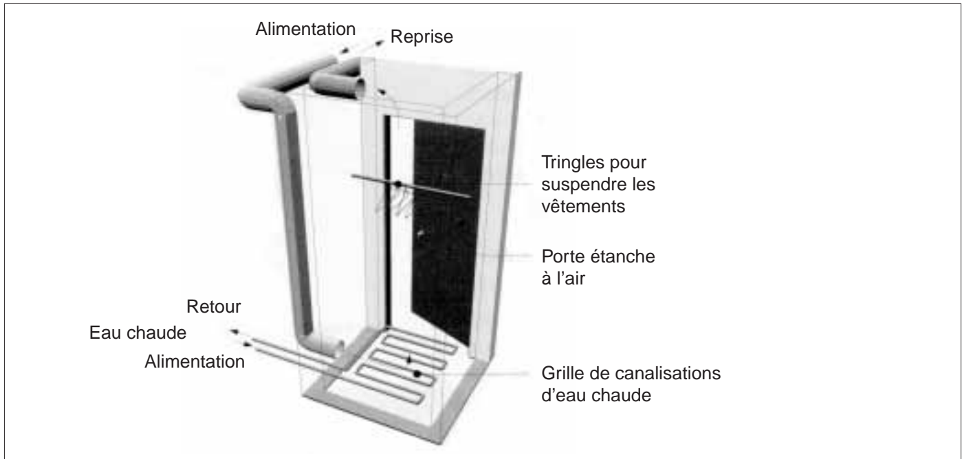
Figure 9 : Penderie de séchage
