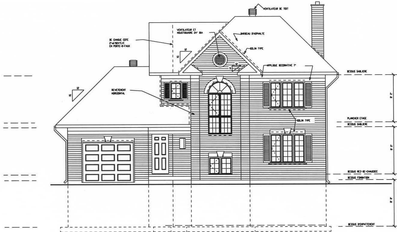
PLAN DE RÉFÉRENCE D'UNE MAISON NOVOCLIMAT
